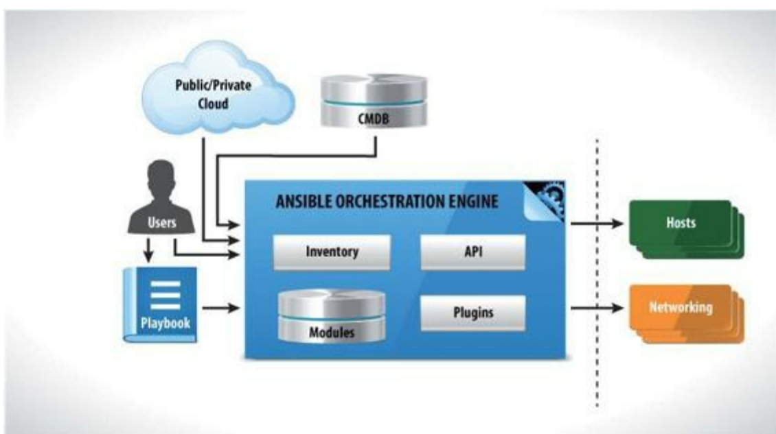
图9-1 Ansible架构图
