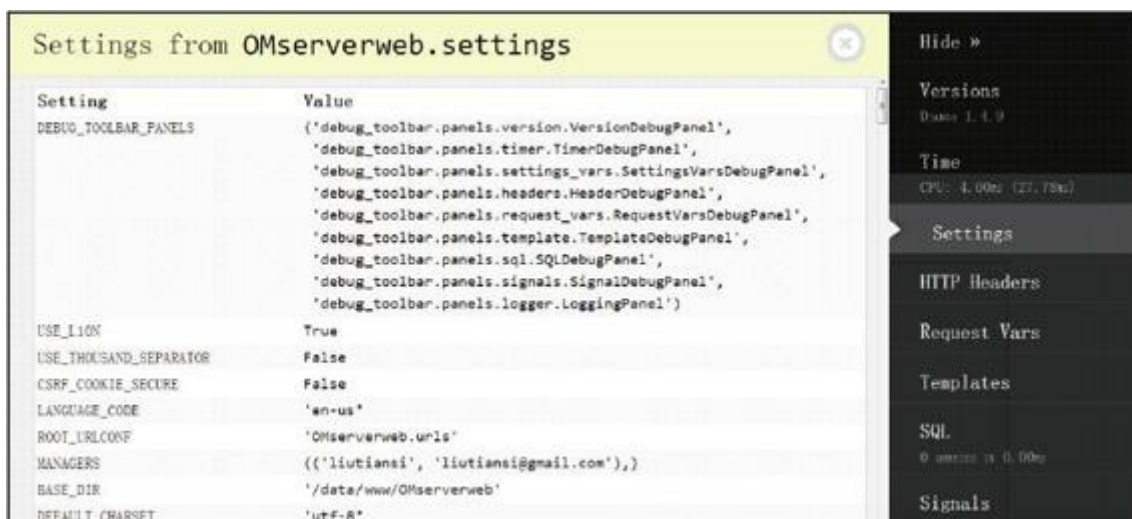
图13-5 debug_toolbar界面
