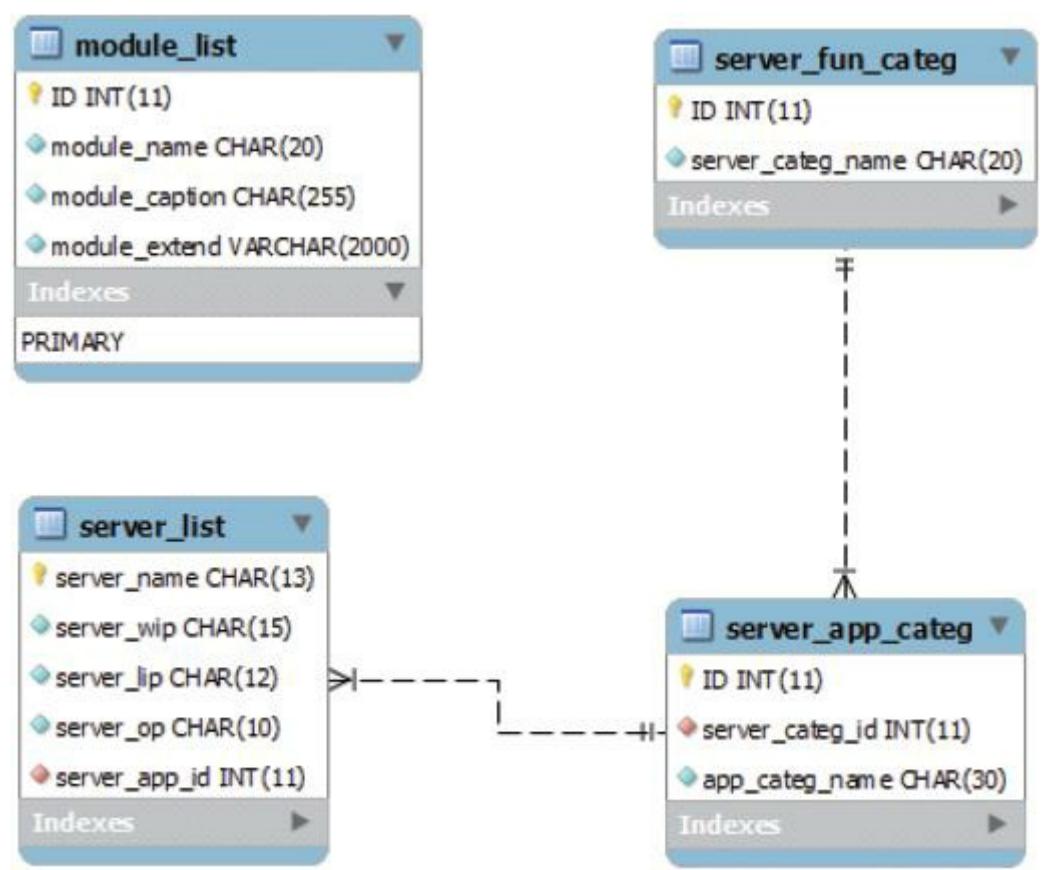
图13-3 数据库模型
