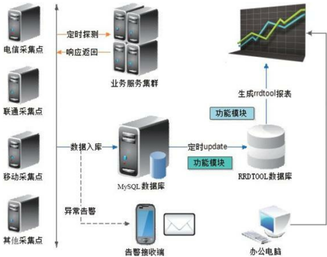
图15-2 系统架构图
