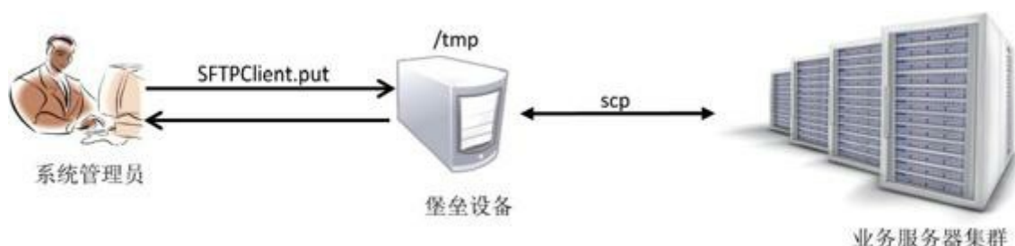
图6-3 堡垒机模式下的文件上传
