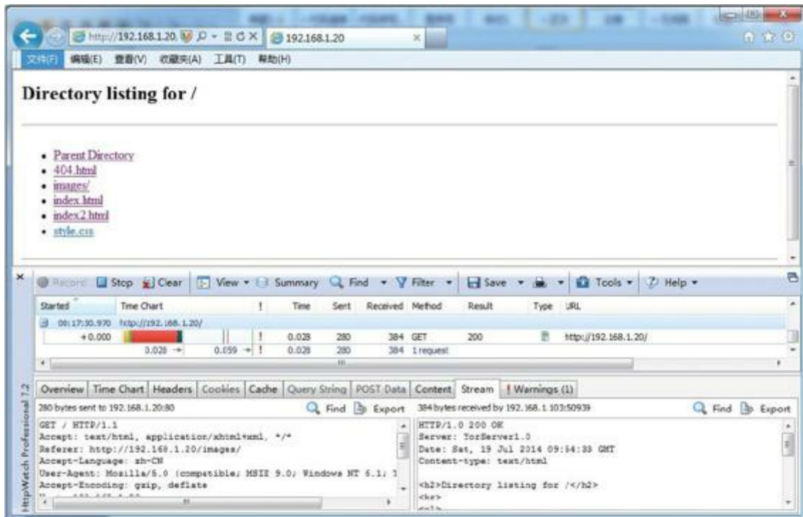
图8-8 目录列表
