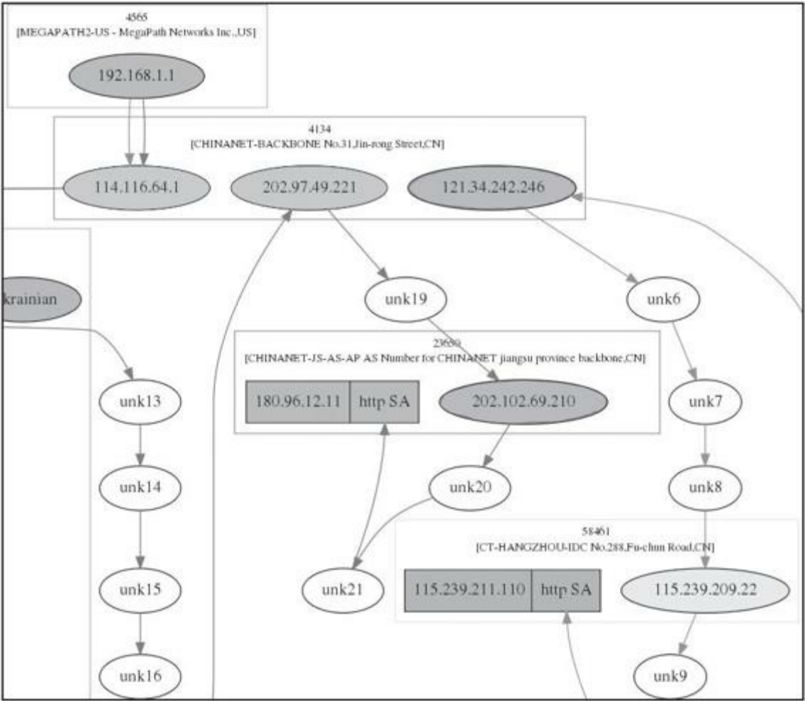
图3-16 路由轨迹图
