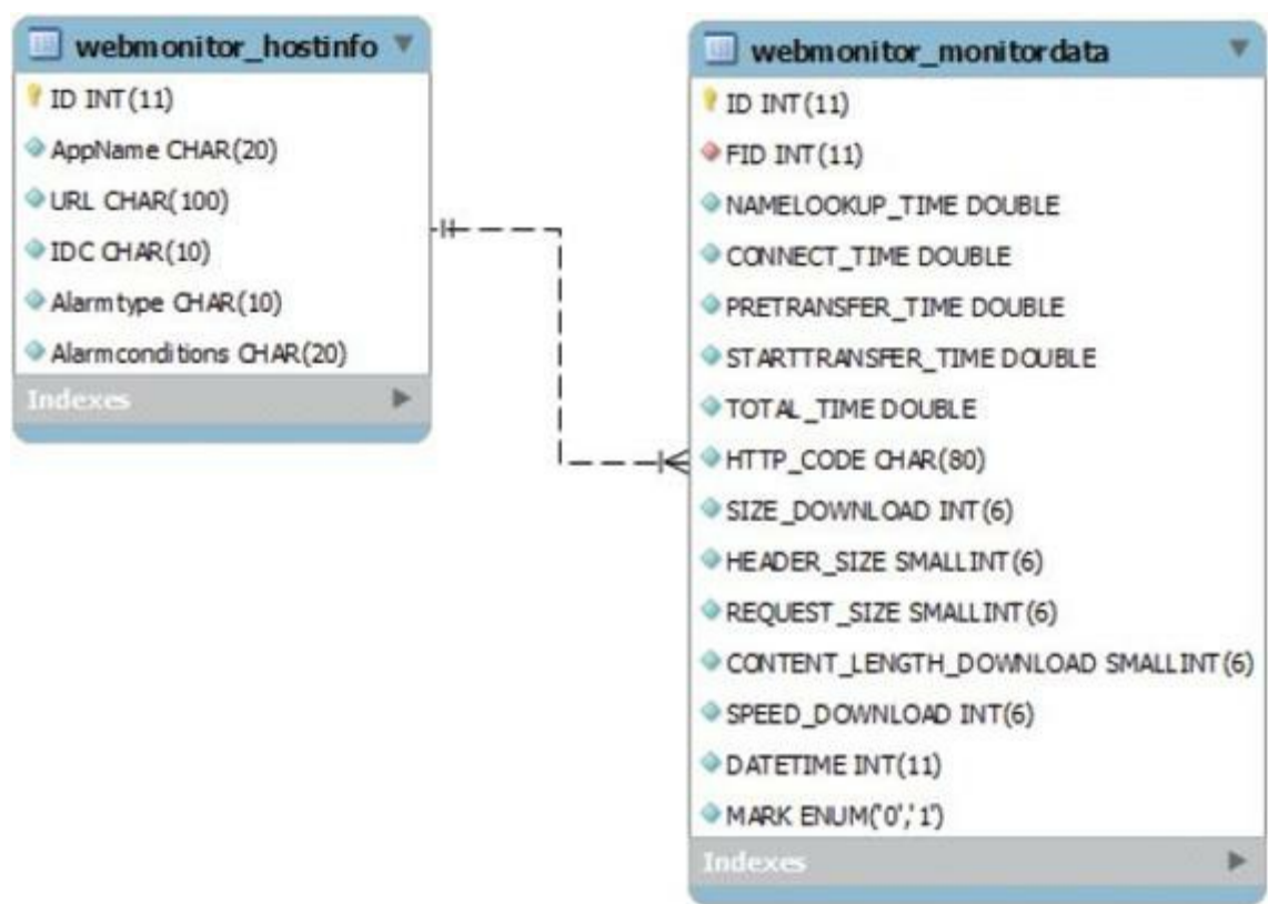
图15-3 系统数据库模型
